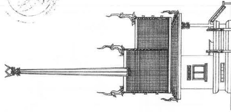
รูปด้านข้าง SCALE 1:125
